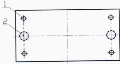
1 - датчики весов, 2 - зона установки образцового динамометра Рисунок 2 - Схема взаимного расположения весовых датчиков и образцового динамометра на платформе весов
