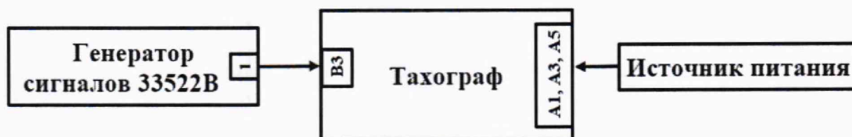
Рисунок 3 – Схема проведения измерений при определении абсолютной инструментальной погрешности измерений скорости по датчику движения
