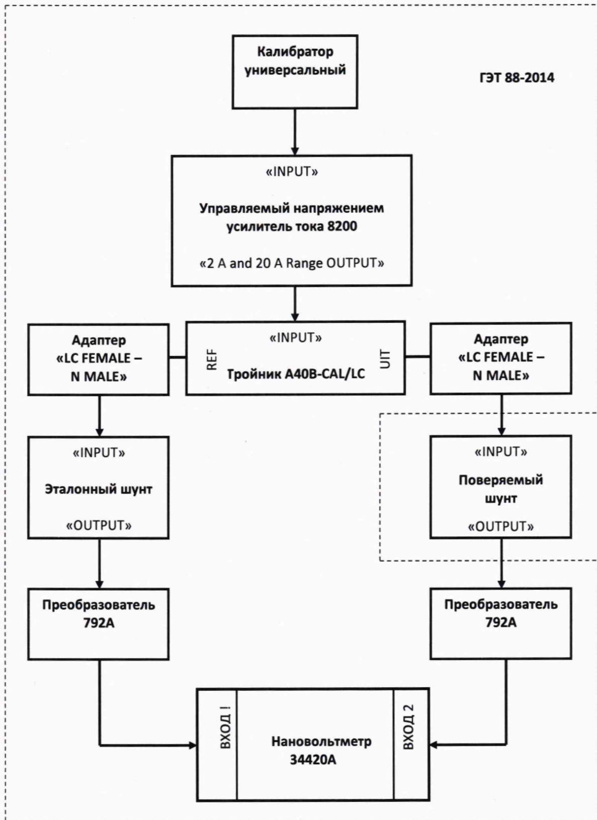
Рисунок 2 Схема соединения приборов при определении метрологических характеристик шунтов переменного тока в диапазоне силы токов св. 2 А и до 20 А включ.
