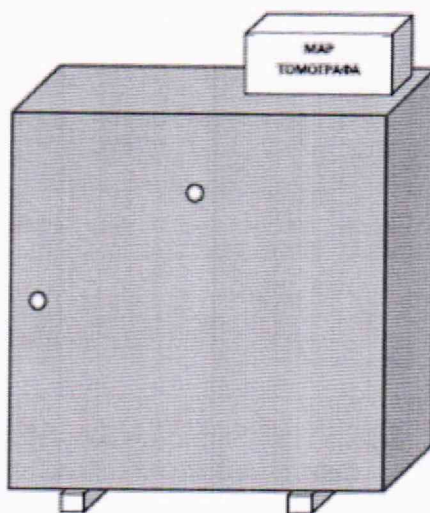
Рисунок 5. Установка MAP томографа на меры МБ3 и МБ4 для измерения толщины 500 мм.
