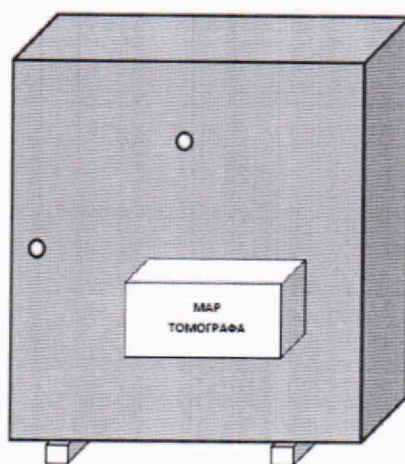
Рисунок 4. Установка MAP томографа на меры МБ3 и МБ4 для измерения толщины 200 мм.
