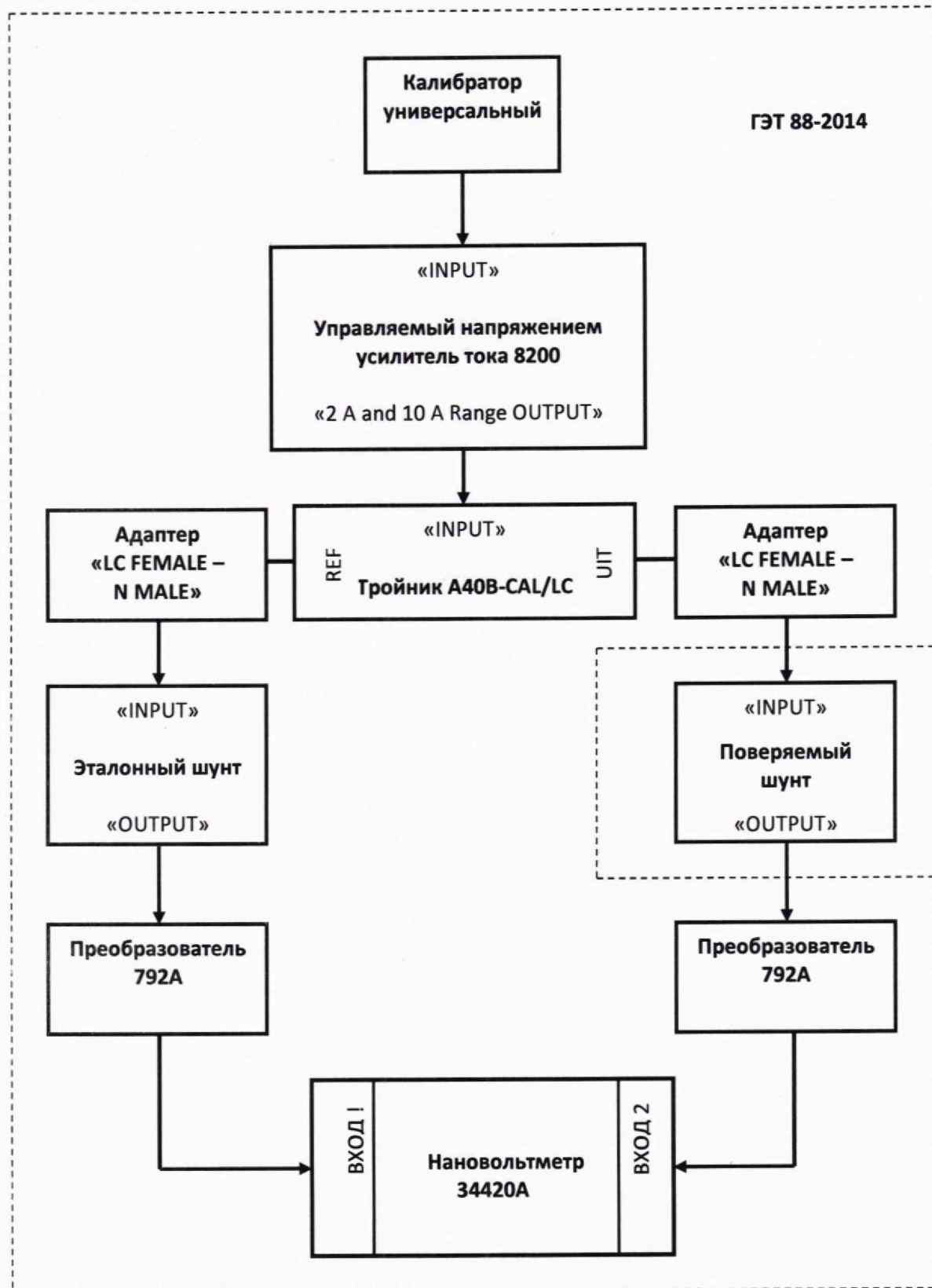
Рисунок 2 Схема соединения приборов при определении метрологических характеристик шунтов переменного тока в диапазоне силы токов св. 2 А и до 10 А включ.
