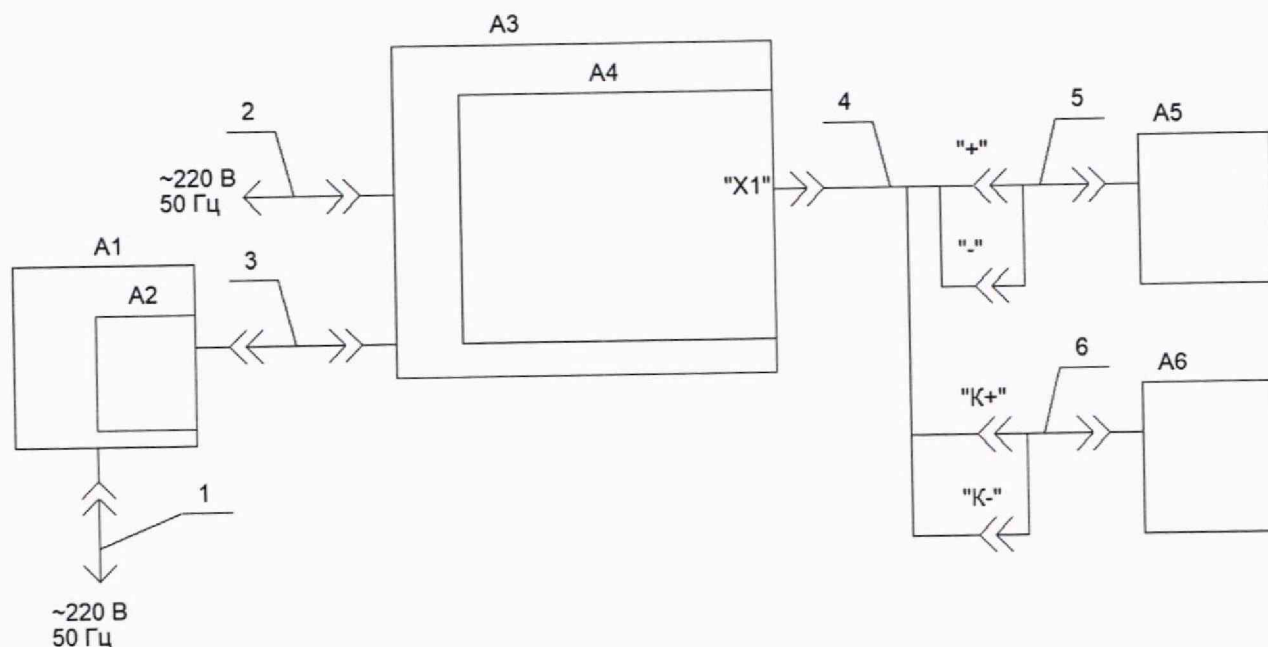
Рисунок 2 – Схема рабочего места,
