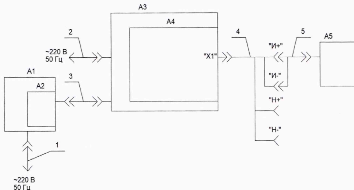
Рисунок 1 – Схема рабочего места,
