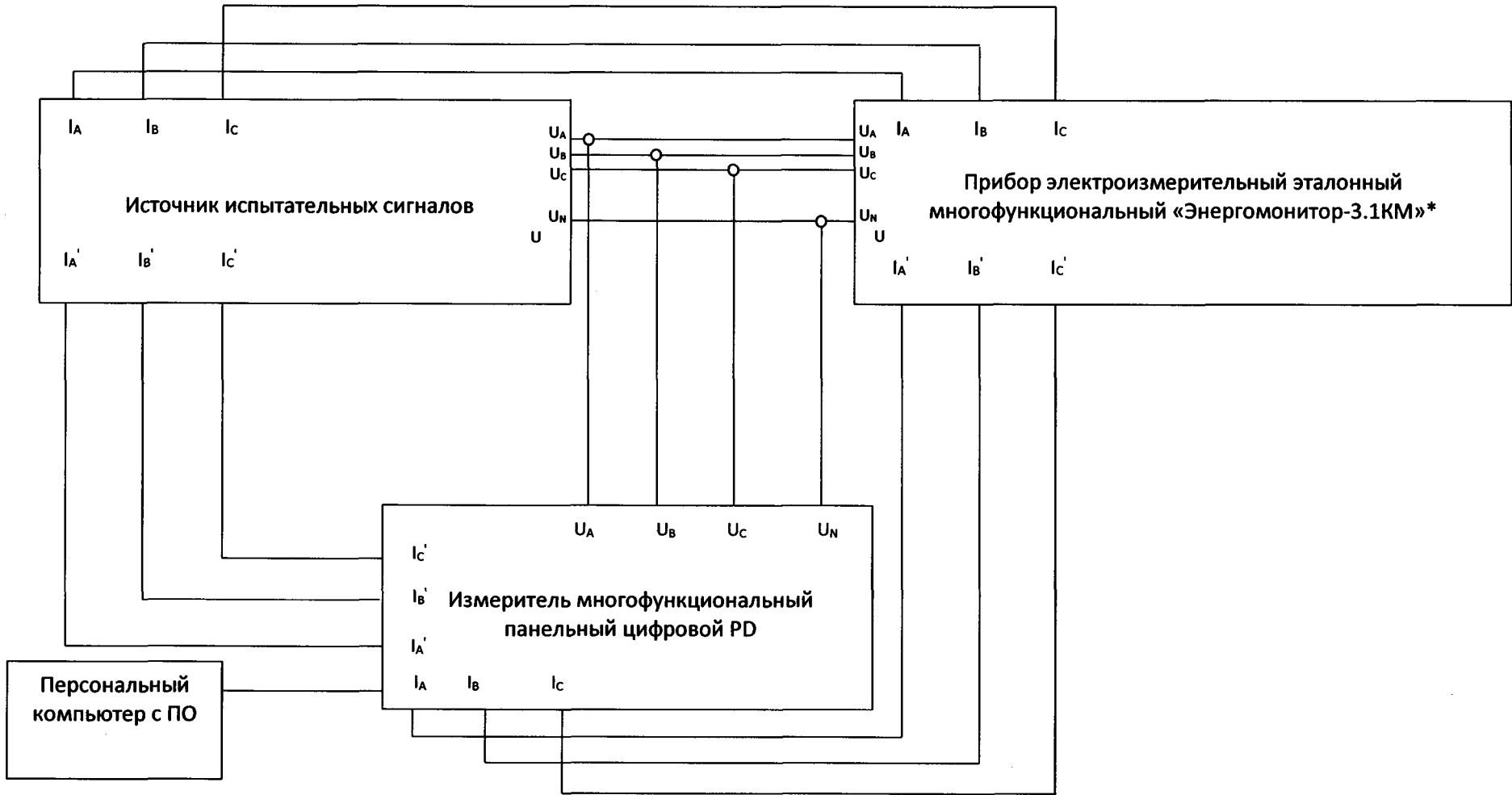
Рисунок 1 – Схема структурная определения метрологических характеристик
