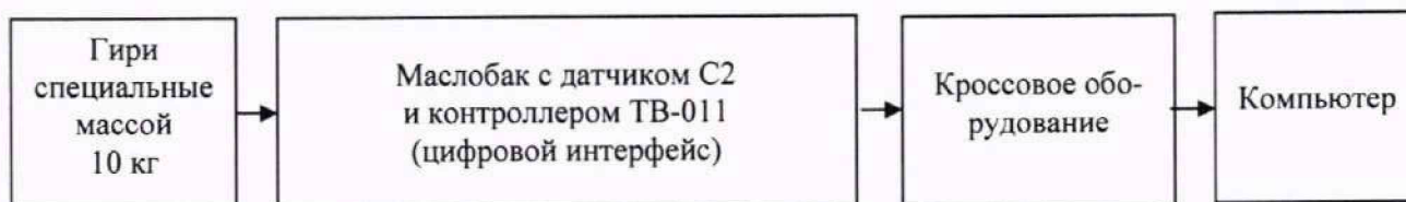
Рисунок 13 - Схема определения метрологических характеристик ИК массы масла
