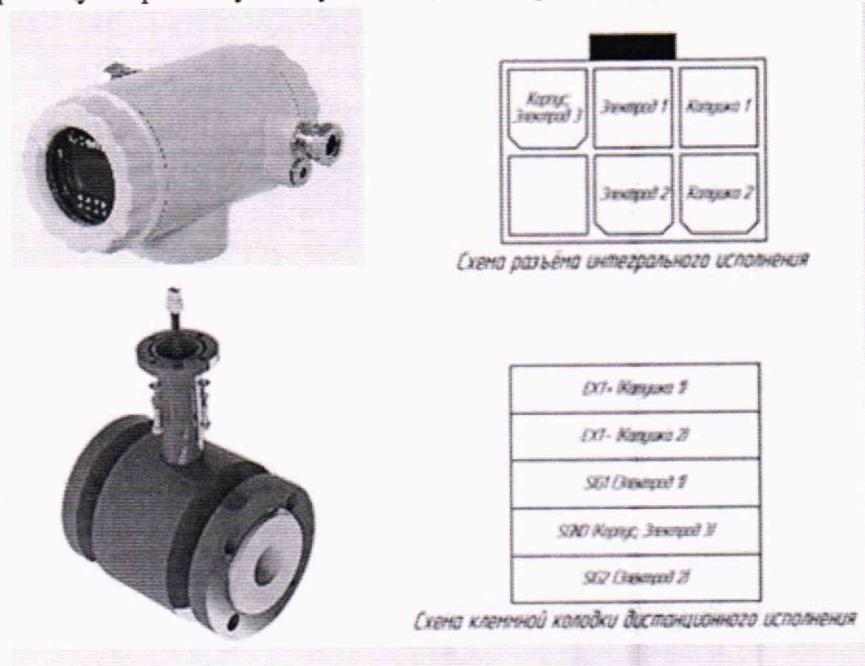
Рисунок 1. Обозначение контактов расходомера Энергия-Э
