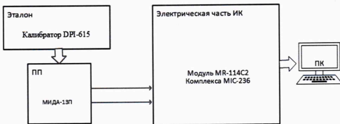
Рисунок 4 – Схема поверки ИК избыточных давлений комплектным способом
