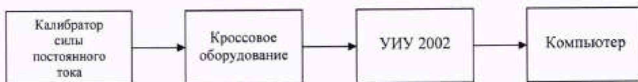
Рисунок 12 - Схема определения метрологических характеристик ИК силы постоянного тока
