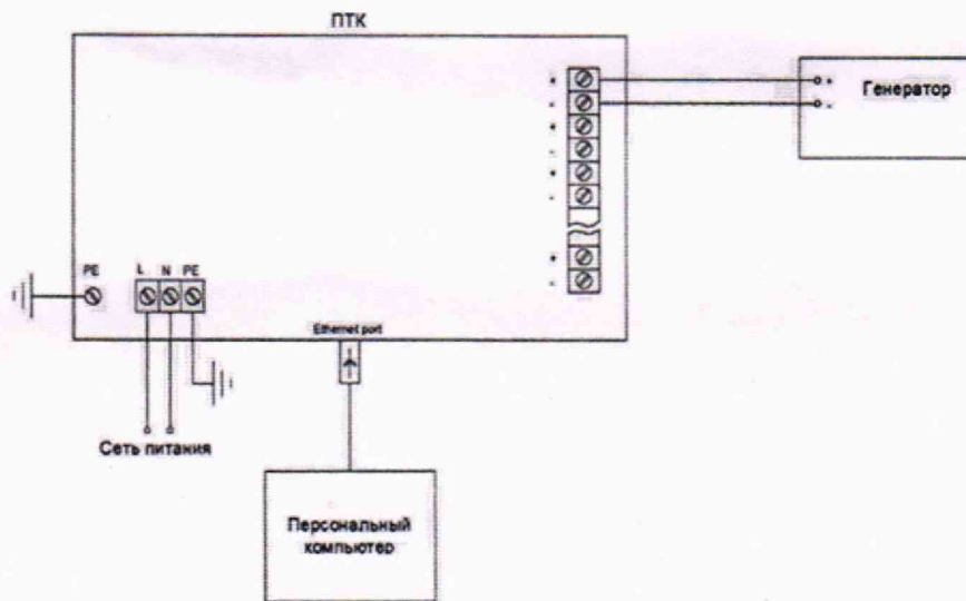
Рисунок 3 – Схема подключений при определении относительной погрешности измерений частоты следования импульсов
