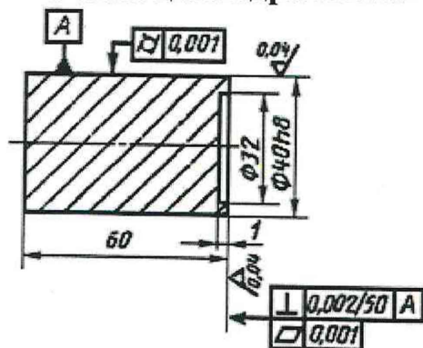
Рисунок Г.1 – Чертеж общего вида ролика цилиндрического Материал сталь У8А по ГОСТ 1435-99 Твердость: 58...61 НРС
