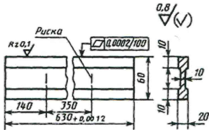
Рисунок А1 – Чертеж контрольного бруска для определения отклонения от прямолинейности измерительных поверхностей угольников модификации УЛП
