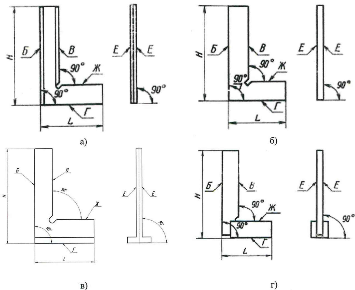
Рисунок Б1 – Обозначение поверхностей угольников поверочных 90^\circ Метроп модификаций: а) УЛП; б) УП; в) УШ модель 1; г) УШ модель 2
