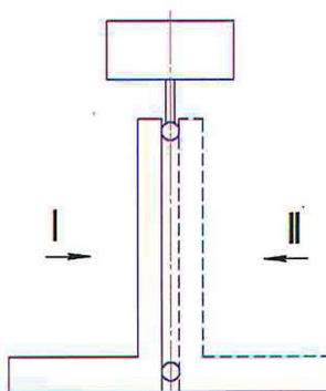
Рисунок 3 – Определение отклонения от перпендикулярности наружной измерительной поверхности к опорной поверхности угольника.
