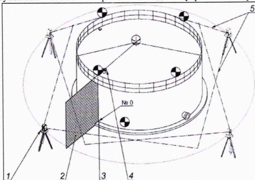
1 - станция сканирования; 2 - плоскость А; 3 - сферическая марка, установленная на ограждении кровли; 4 - точка измерения базовой высоты;
