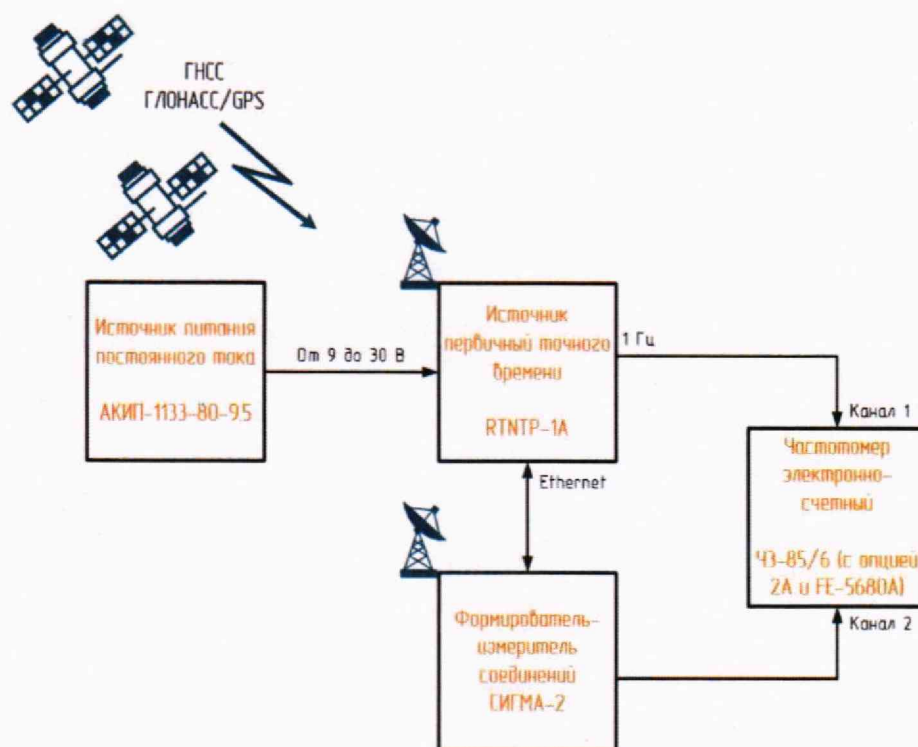
Рисунок 1 – Схема измерений для поверки
