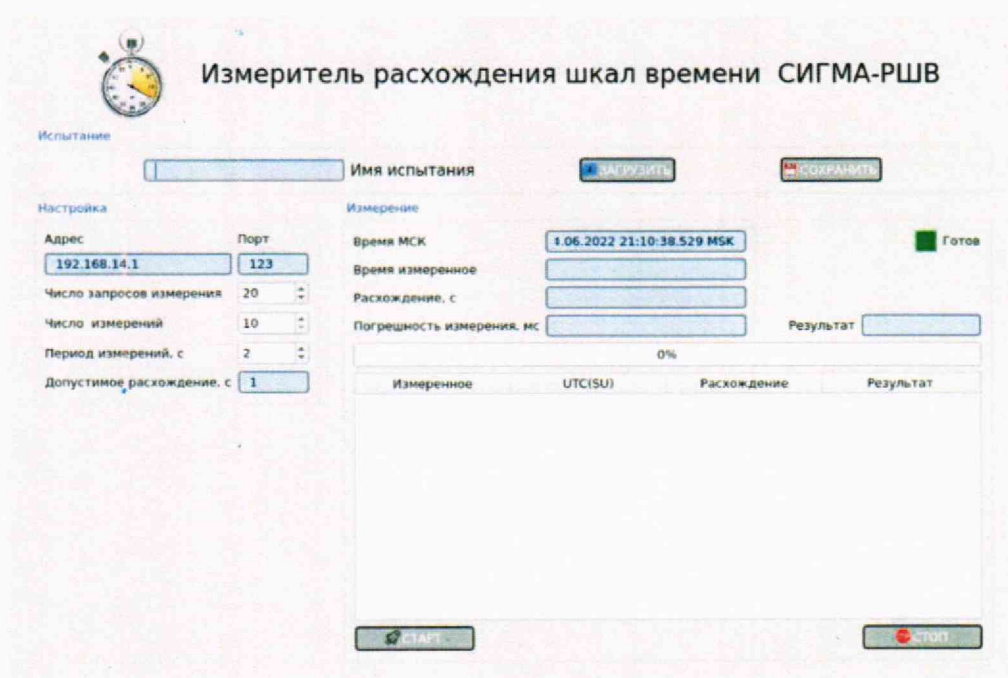
Рисунок 9. Основное окно подпрограммы СИГМА-РШВ
