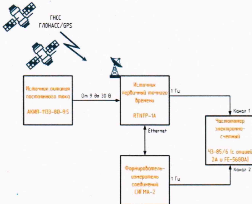
Рисунок 7. Схема измерений при определении абсолютной погрешности синхронизации формируемой шкалы времени с национальной шкалой времени UTC(SU) по протоколу NTP на интерфейсе Ethernet
