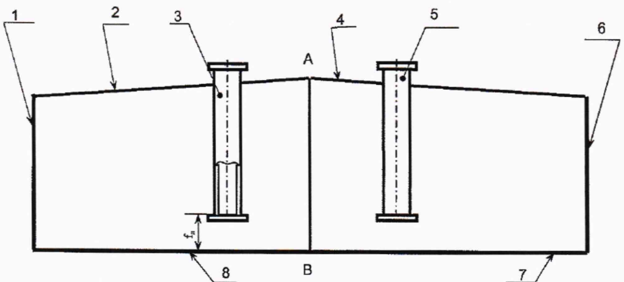
1, 6 – боковые переборки; 2, 4 – палуба судна; 3, 5 – измерительные трубы; 7, 8 – днища танков f_{л} – высота точки касания дна измерительной трубы грузом рулетки; AB – диаметральной плоскость судна
