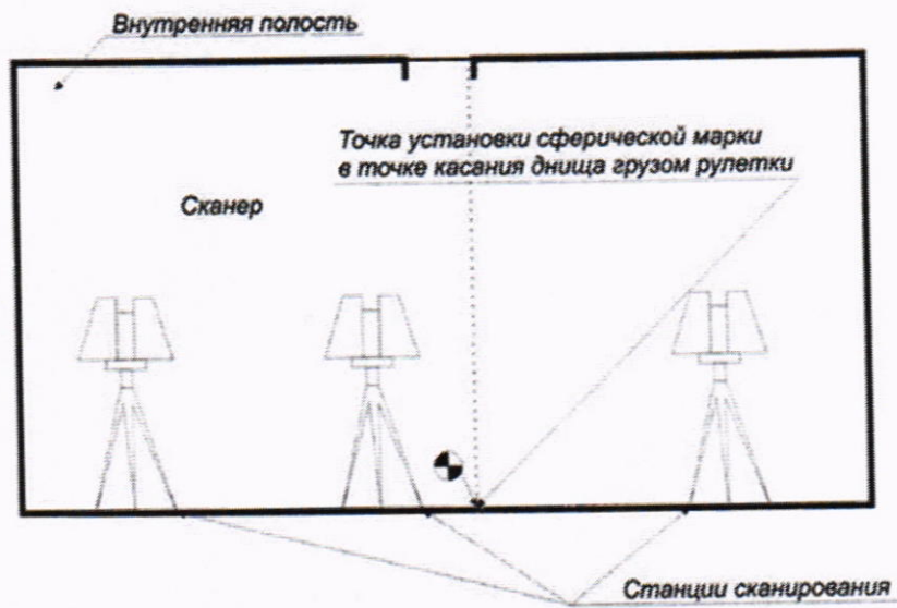
Рисунок А.2 - Схема сканирования внутренней полости резервуара
