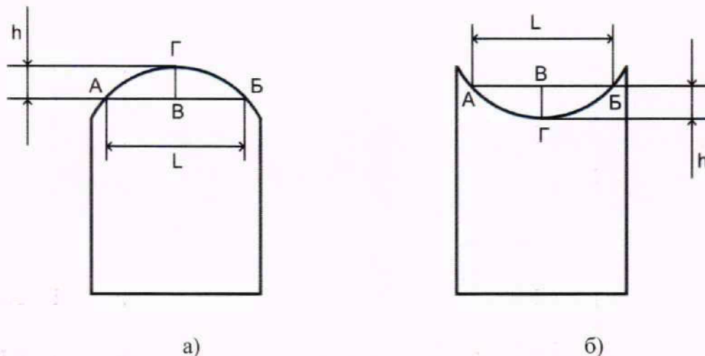
Рисунок 11 – Измерения радиуса
