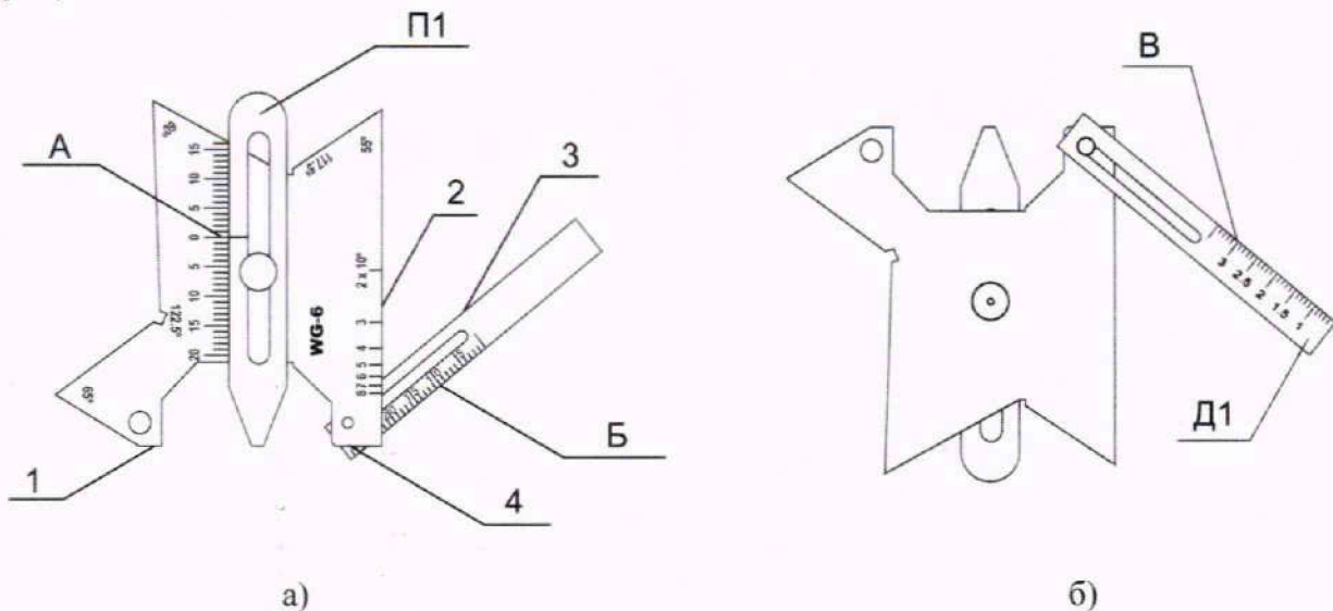
Рисунок 5 - Общий вид шаблонов сварщика универсальных WG, исполнение WG-6
