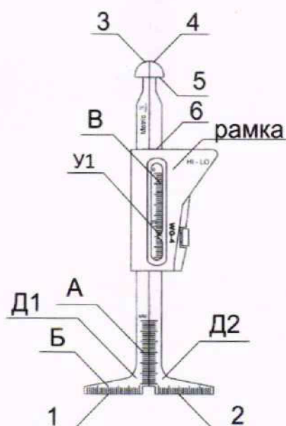
Рисунок 2 – Общий вид шаблонов сварщика универсальных WG, исполнение WG-4 А, Б, В – шкалы; 1 - 6 – поверхности; Д1 – первый измерительный движок; Д2 – второй измерительный движок; У1 – указатель шкалы В
