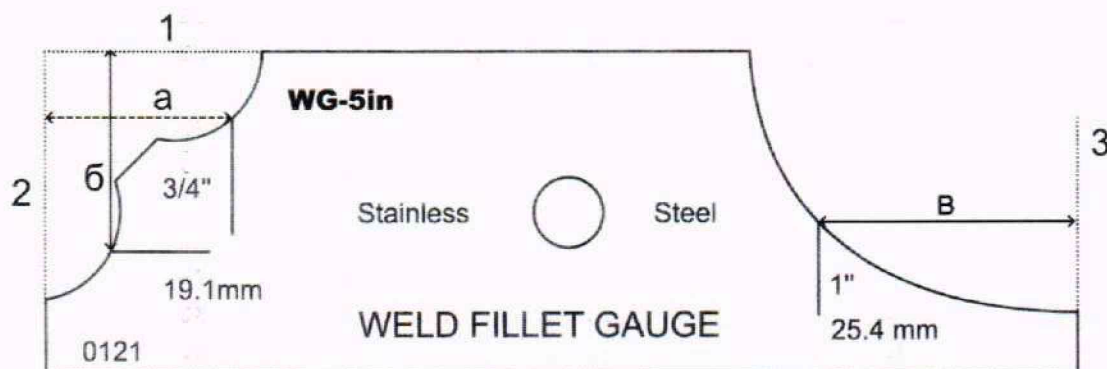
Рисунок 4 - Определение толщины и катета углового шва
