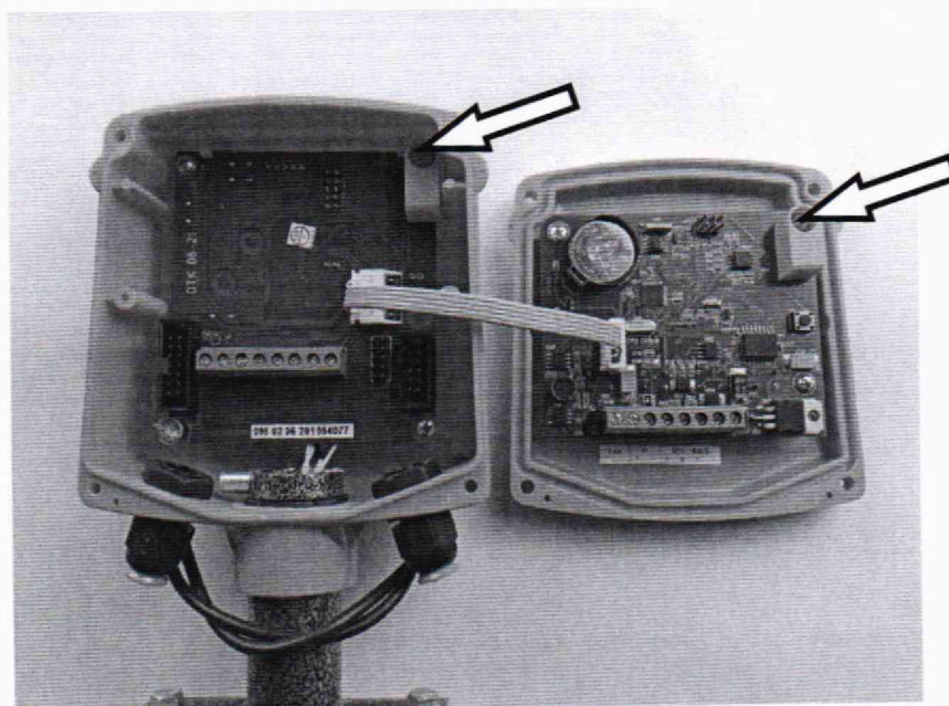
Рисунок А.1 – Обозначение мест нанесения знаков поверки
