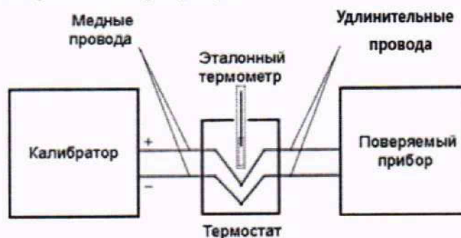
Рисунок 1 – Схема подключения
