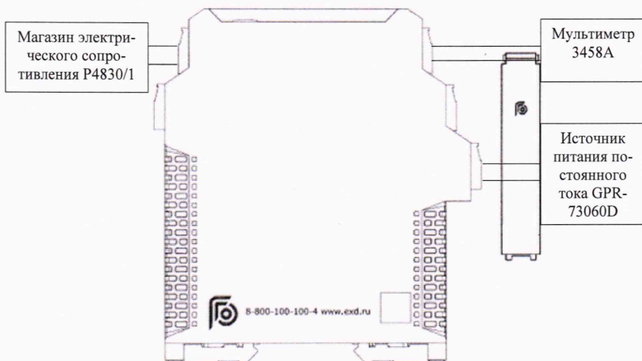
Рисунок 2 – Схема подключения для определения основной приведенной к диапазону выходного сигнала погрешности преобразований входного сигнала от термопреобразователей сопротивления по ГОСТ 6651-2009 в выходной сигнал
