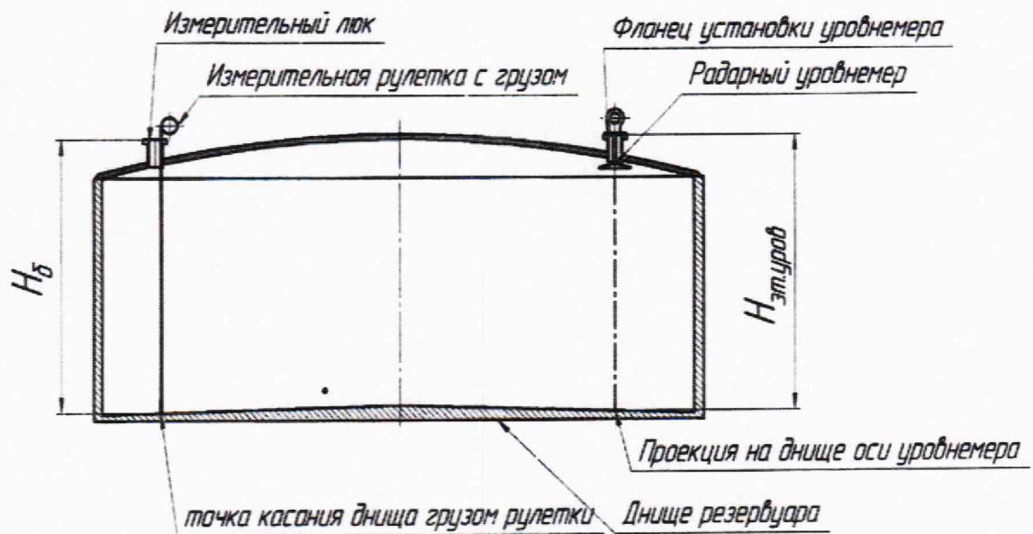
Рисунок А.1 – Схема измерения базовой высоты резервуара и эталонного расстояния урбнемера
