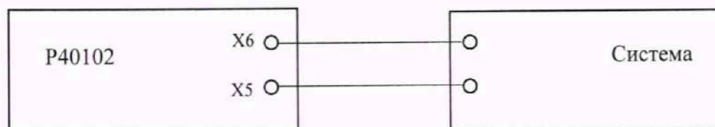
Рисунок 9 – Схема подключения для определения относительной погрешности измерений электрического сопротивления изоляции с использованием P40102
