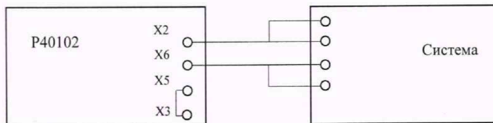
Рисунок 7 – Схема подключения для определения относительной погрешности измерений электрического сопротивления постоянному току по четырехпроводной схеме с использованием P40102
