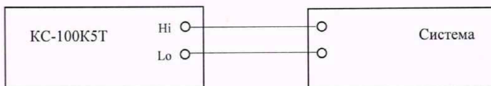
Рисунок 8 – Схема подключения для определения относительной погрешности измерений электрического сопротивления изоляции с использованием КС-100К5Т
