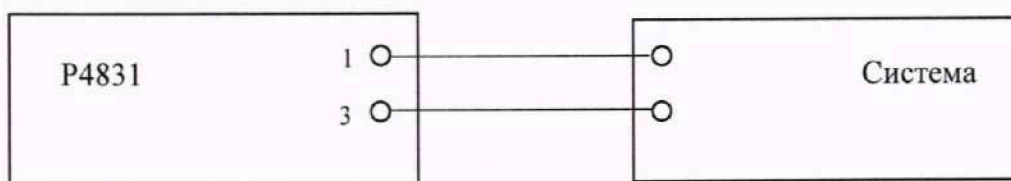
Рисунок 4 – Схема подключения для определения относительной погрешности измерений электрического сопротивления постоянному току по двухпроводной схеме и электрического сопротивления изоляции с использованием Р4831
