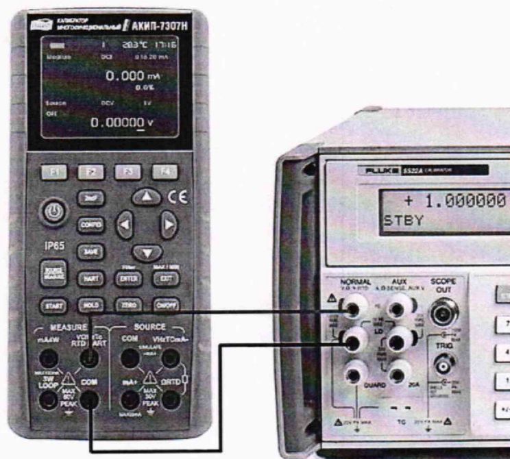
Рисунок 1 – Схема соединения приборов при определении погрешности измерения напряжения постоянного тока и частоты.
