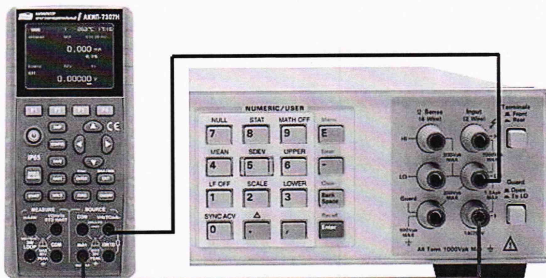
Рисунок 6 – Схема соединения приборов при определении погрешности воспроизведения силы постоянного тока.
