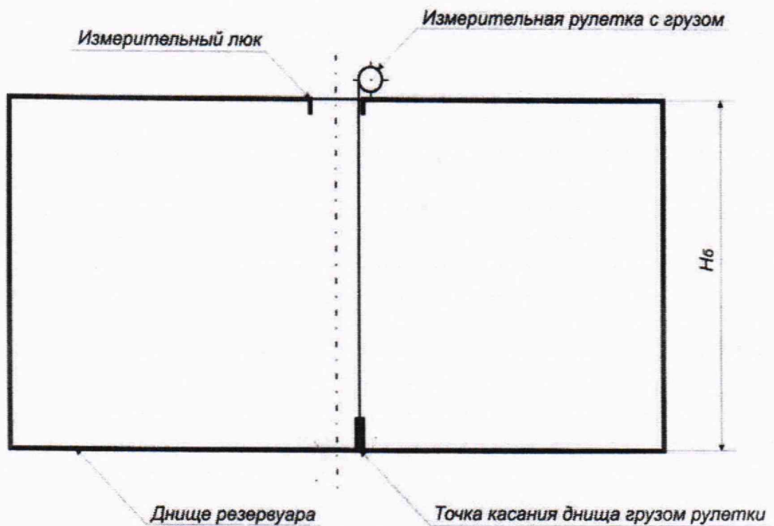
Рисунок А.1 – Схема измерения базовой высоты резервуара и эталонного расстояния уровня
