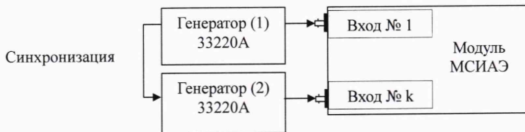
Рисунок А3 – Схема подключения приборов для проверки диапазона и определения абсолютной погрешности измерений разности времени поступления сигнала на каналы
