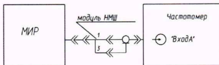
Рисунок 2 – Схема проверки при определении относительной погрешности воспроизведения опорной частоты
