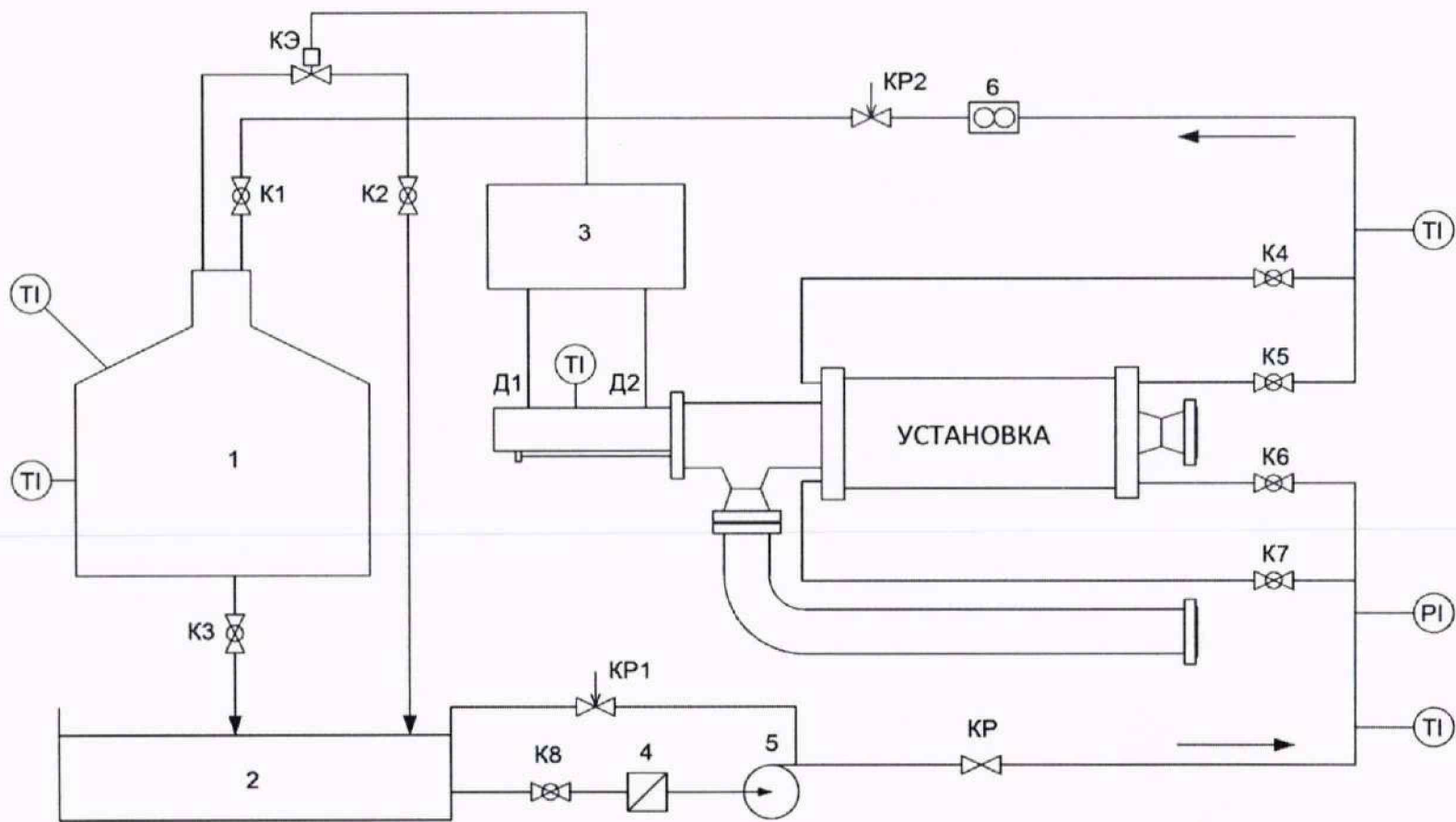
Схема А – Принципиальная схема соединений поверяемой установки и средств поверки с применением мерника с верхним заполнением 1 – мерник; 2 – емкость-хранилище; 3 – панель управления установкой; 4 – фильтр; 5 – насос; 6 – расходомер; Д1, Д2 – детекторы; К1 – К8 – запорная арматура; КР – кран регулирующий; КЭ – клапан электромагнитный; УСТАНОВКА – поверочная установка; Тl – термометр; Рl – манометр
