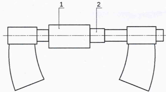
1 – мера длины концевая; 2 – динамометр
