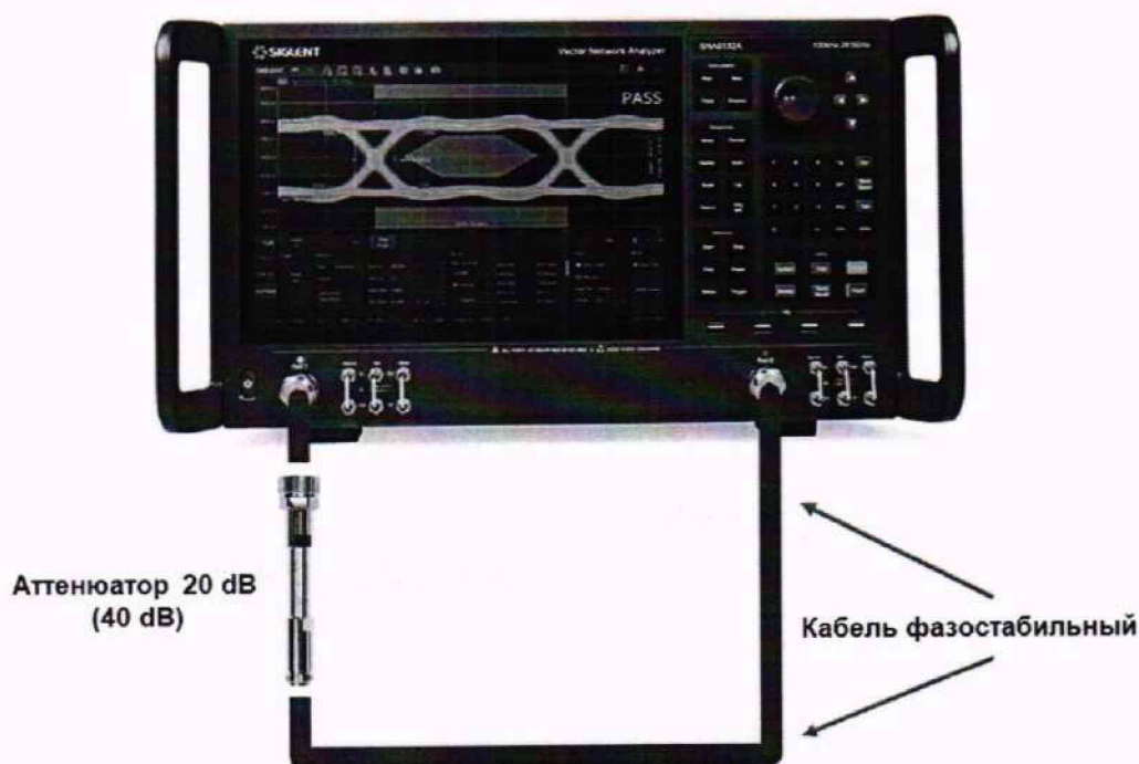
Рисунок 6 – Схема соединения приборов для определения погрешности измерения модуля и фазы коэффициента передачи
