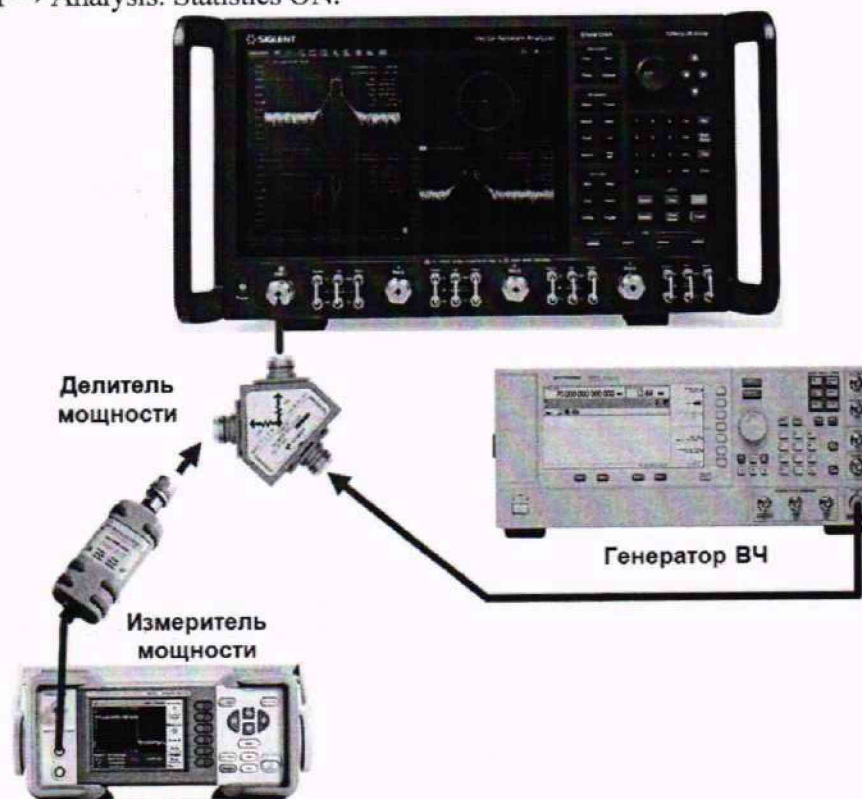
Рисунок 3 – Схема соединения приборов для определения абсолютной погрешности измерений уровня мощности
