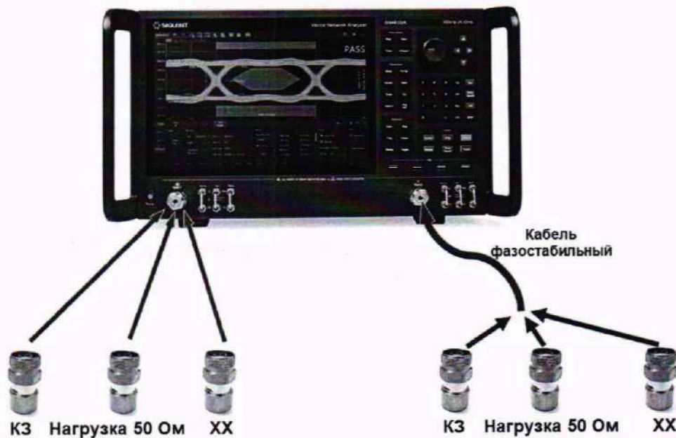
Рисунок 5 – Схема соединения приборов для определения погрешности измерения модуля и фазы коэффициента отражения
