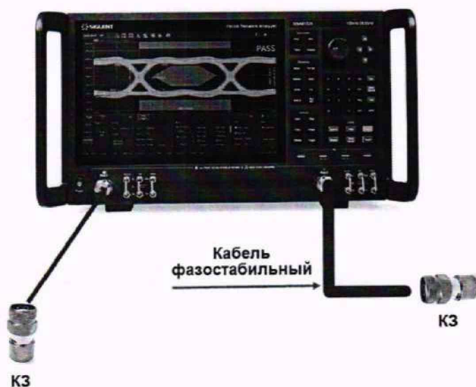
Рисунок 4 – Схема соединения приборов для измерения среднеквадратического отклонения шумов измерительного тракта
