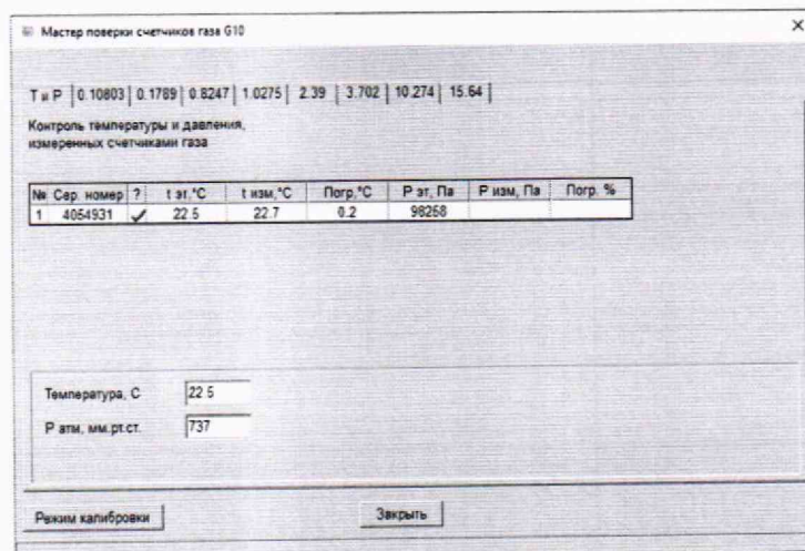
Рисунок 2 – Поверка канала измерения температуры по программе FlowTune.exe
