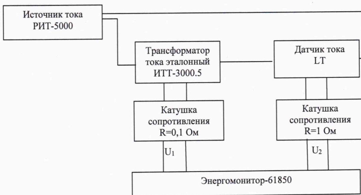
Рисунок 1 - Схема проверки на переменном токе
