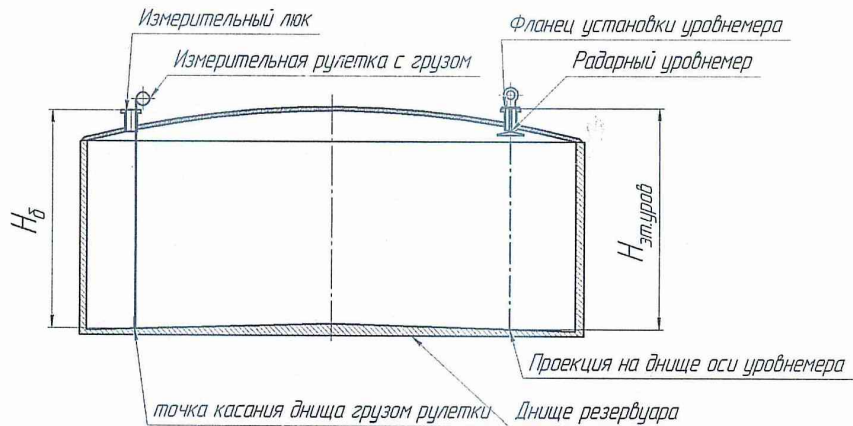
Рисунок А.1 – Схема измерения базовой высоты резервуара и эталонного расстояния уронемера
