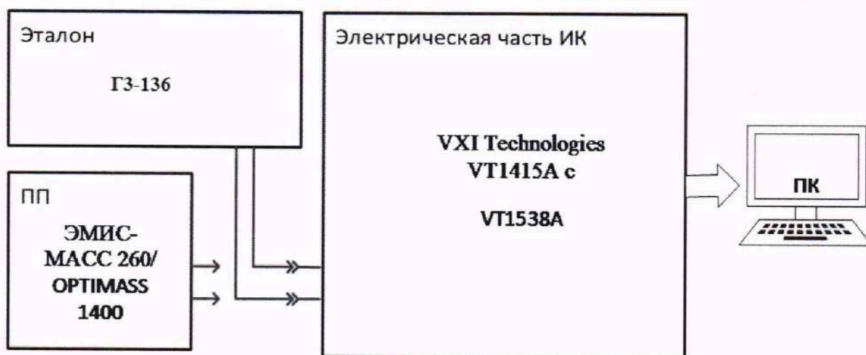
Рисунок 1 – Схема поверки ИК МИРТ
