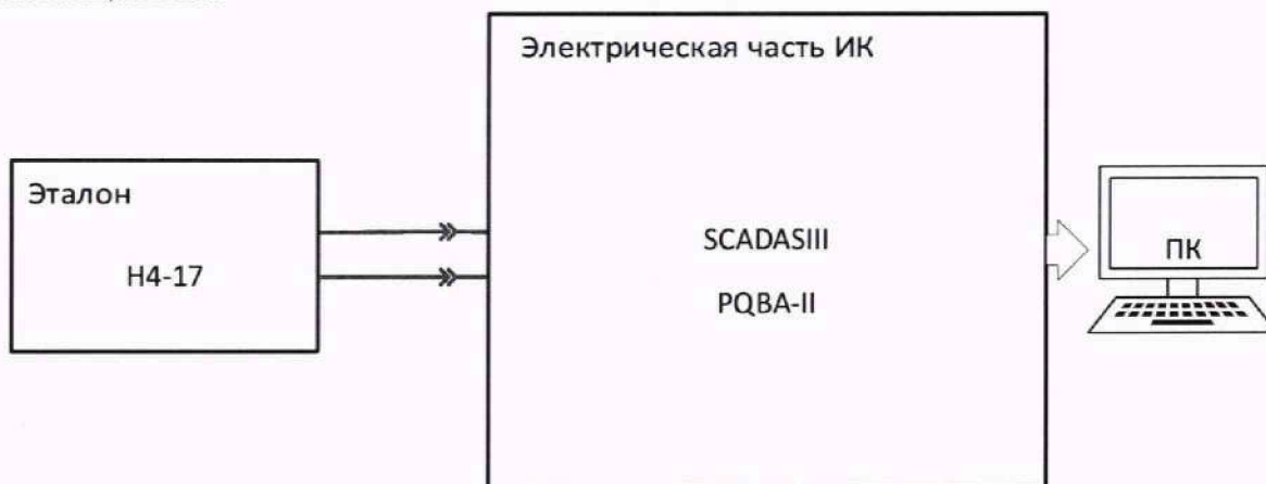
Рисунок 13 – Схема поверки ИК напряжения тензодатчиков
