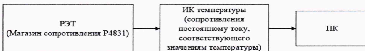
Рисунок 4 - Схема поверки ИК температуры (сопротивления постоянному току, соответствующего значениям температуры), РЭТ магазин сопротивления Р4831
