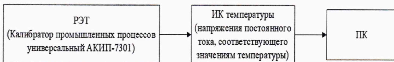
Рисунок 6 - Схема поверки ИК температуры (напряжения постоянного тока, соответствующего значениям температуры), РЭТ калибратор промышленных процессов универсальный АКПП-7301
