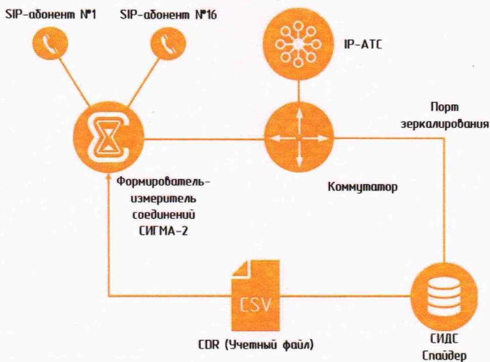
Рисунок 2 – Схема поверки СИДС
