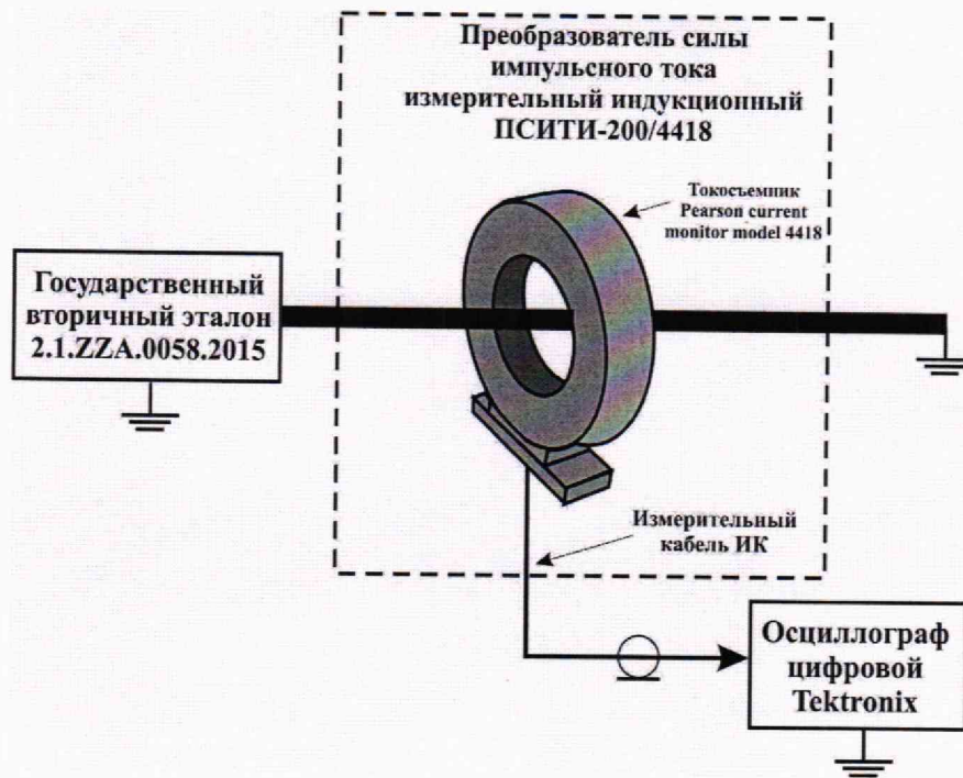
Рисунок 1 – Схема соединений при проведении опробования преобразователя и проверки его метрологических характеристик
