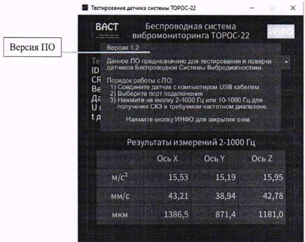
Рисунок 2. Версия ПО
