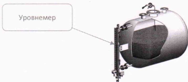
Рисунок 1 - Проверка уровнемера без демонтажа по месту эксплуатации
