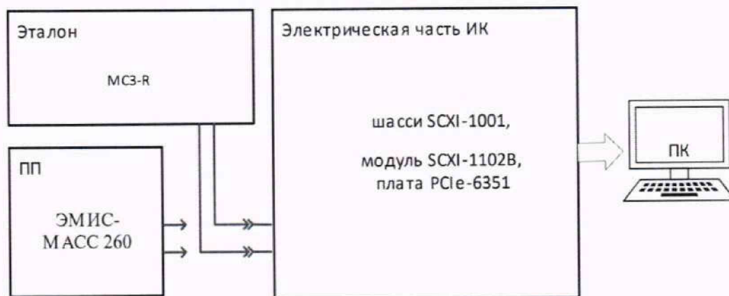
Рисунок 8 – Схема поверки ИК массового расхода топлива
