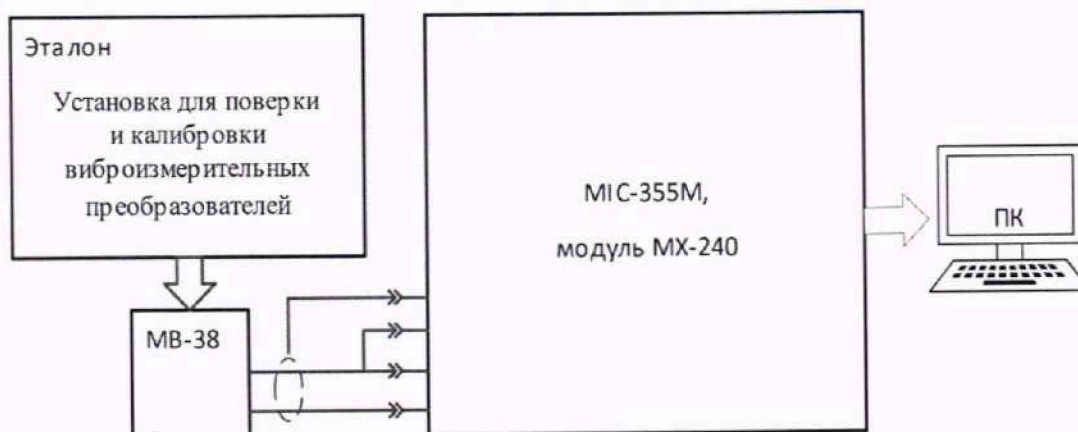
Рисунок 11 – Схема проверки ИК амплитуды виброскорости корпусов ГТД по первым гармоникам роторов
