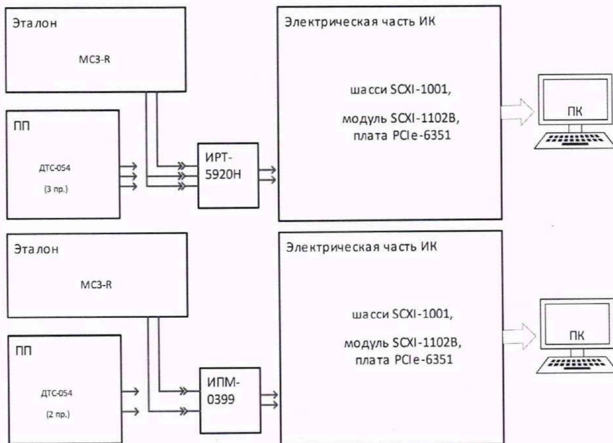
Рисунок 3 – Схемы поверки ИК температур газообразных и жидких сред поэлементным способом
