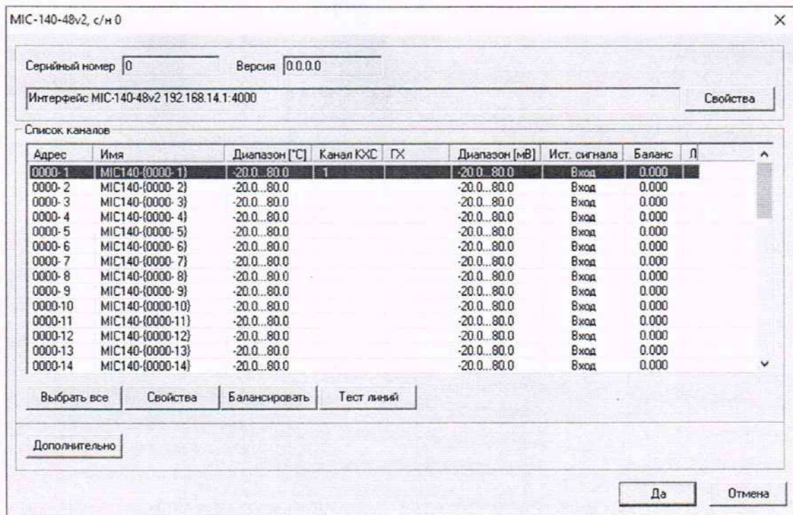
Рисунок Д4 – Окно «Настройка аппаратной части» для МИС-140 после отключения градуировочной характеристики для канала 1
