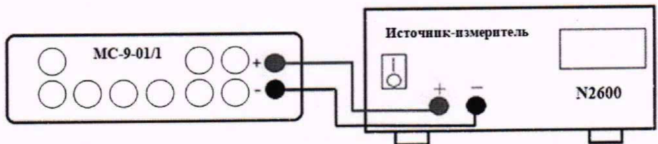
Рисунок 2 – Структурная схема соединения приборов
