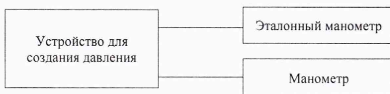
Рисунок 1 – Схема подключений для опробования манометра и определения приведенной к верхнему пределу диапазона измерений основной погрешности измерений разности давлений и вариации показаний манометра
