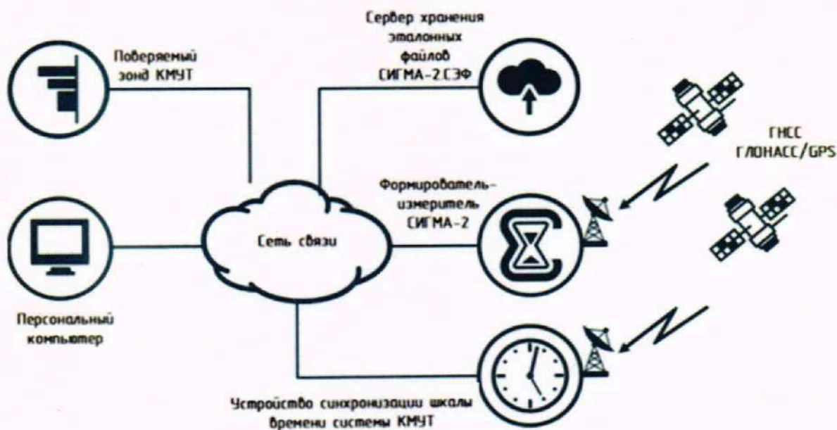
Рисунок 7 – Схема измерений при поверке зонда КМУТ
