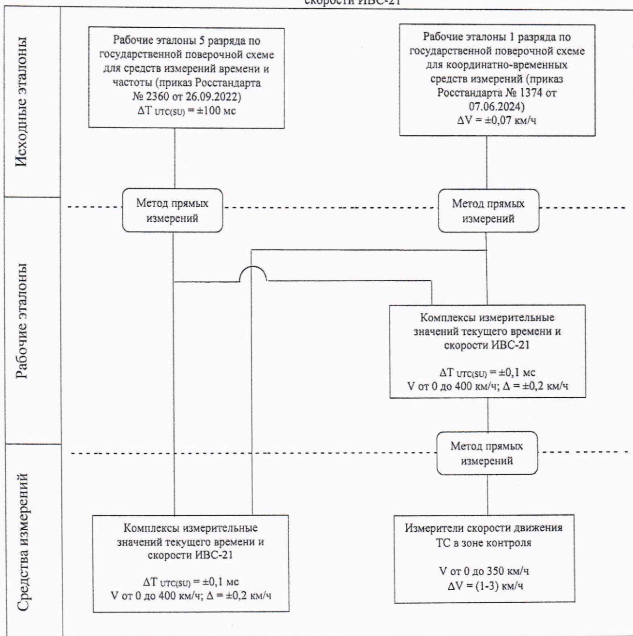
Локальная поверочная схема для комплексов измерительных значений текущего времени и скорости ИВС-21
