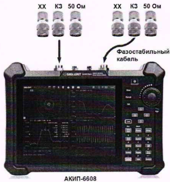
Рисунок 5 – Схема соединения приборов для определения погрешности измерения модуля и фазы коэффициента отражения
