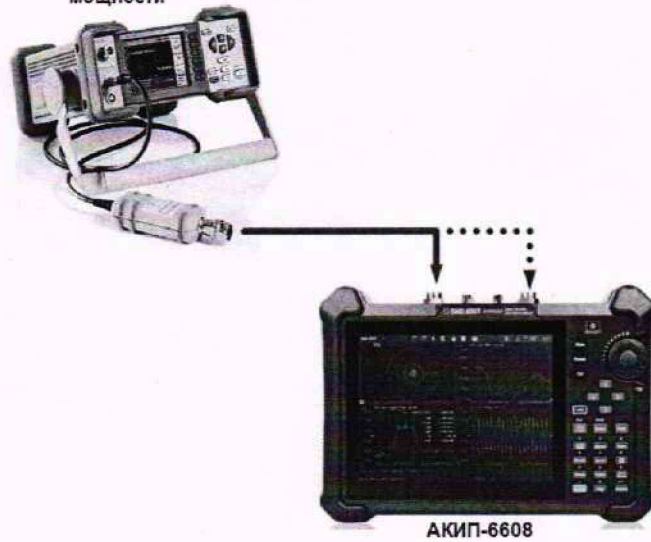
Рисунок 2 – Схема соединения приборов для определения диапазона установки уровня выходной мощности и абсолютной погрешности установки уровня мощности
