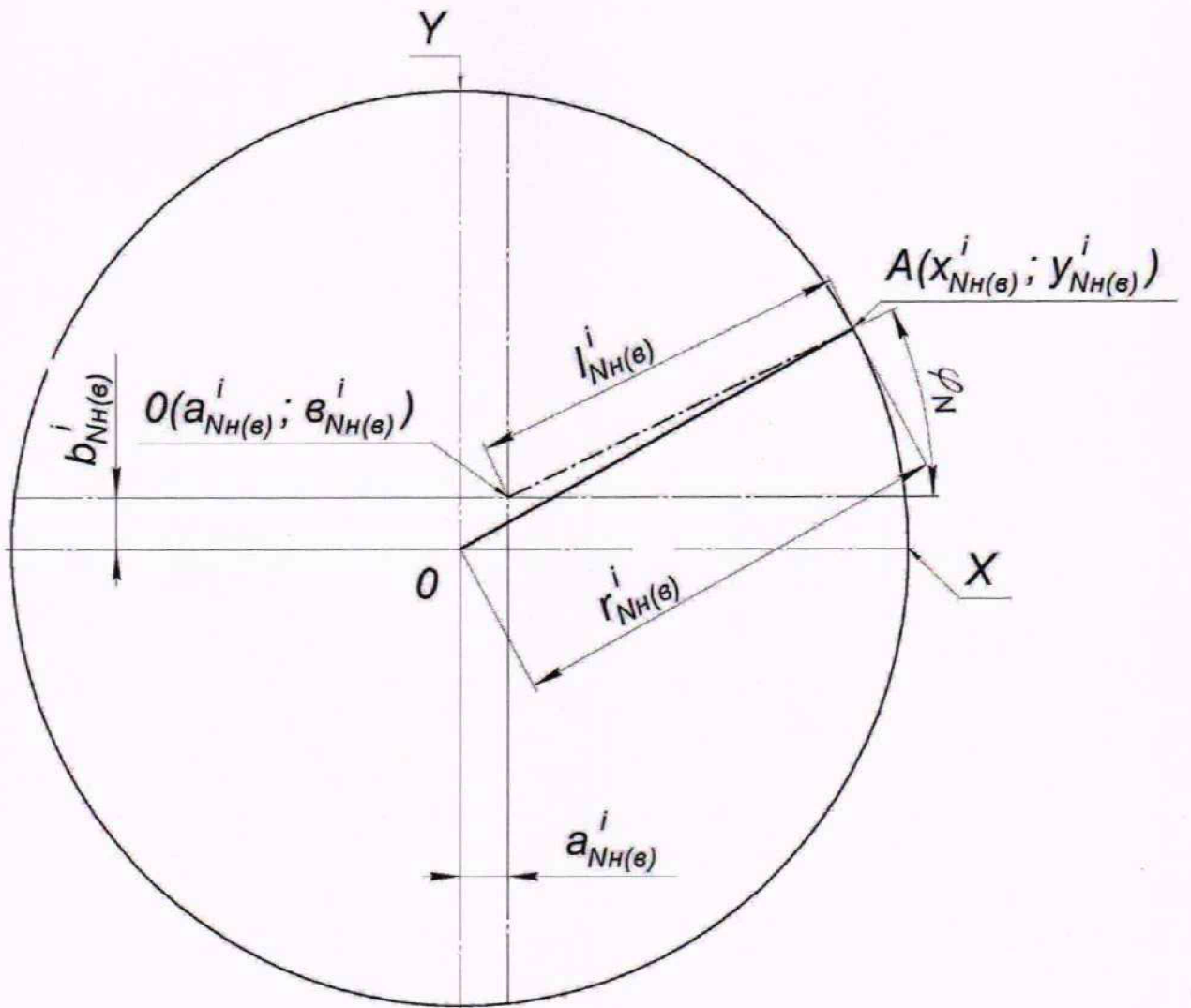
Рисунок Д.2 – Параметры измерений радиуса r_{NH(\epsilon)}^i i -го пояса при j -ом измерении в нижнем (верхнем) сечении
