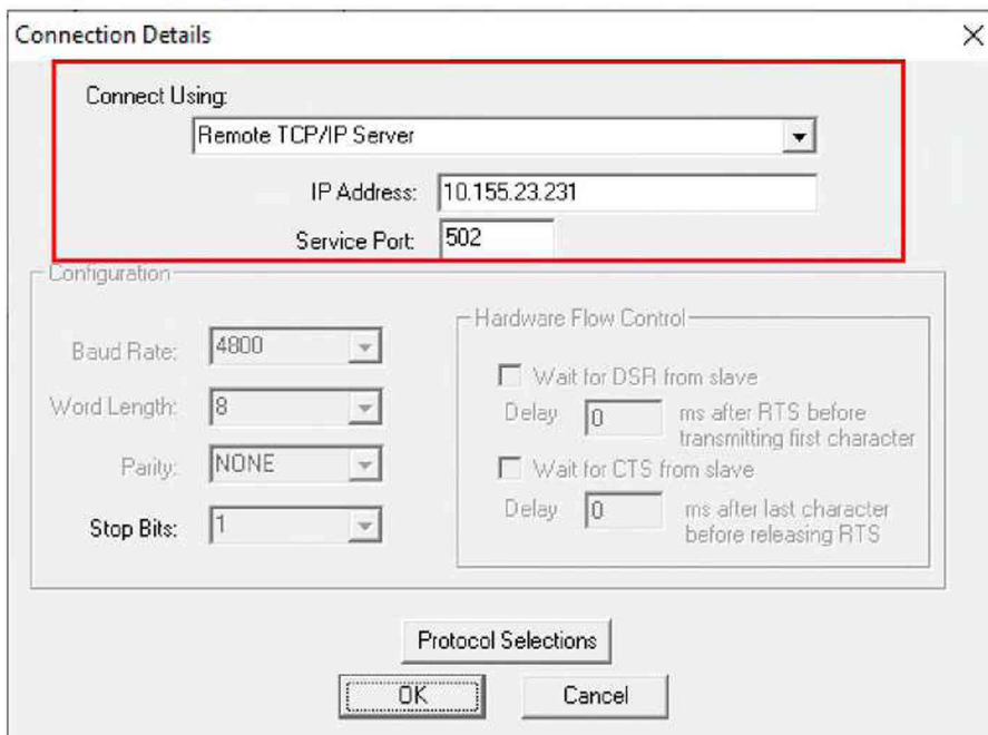
Рисунок 5 – Окно настроек соединения с контроллером
