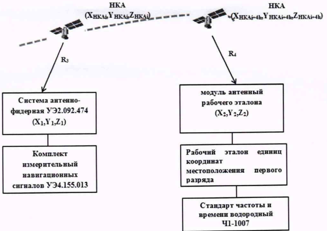
Рисунок 2 - Схема проведения измерений при определении абсолютной систематической погрешности измерений беззапросной дальности в случае размещения изделия и эталона на местах их эксплуатации
